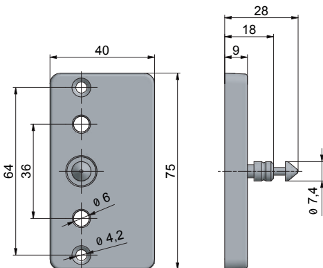
Locking pin SD type C / Schließdorn SD Typ C
